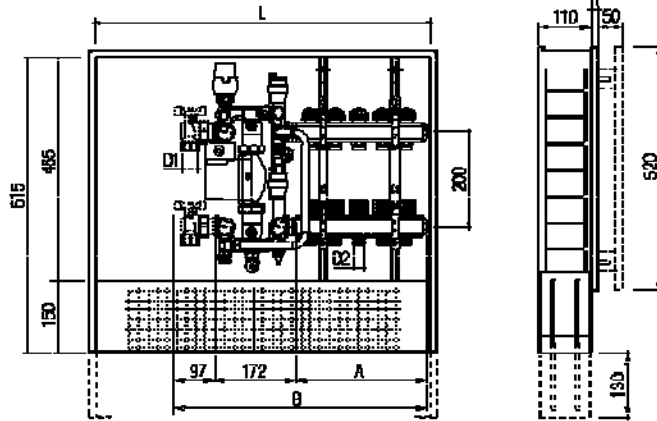
FLOOR CONTROLLER (B) Bassa / Low / Baja Basse / Basse / المنخفض
